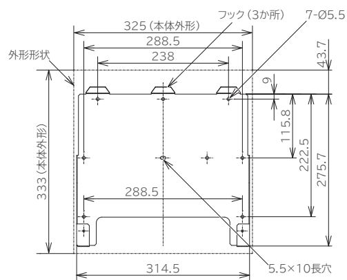
取付板寸法図
