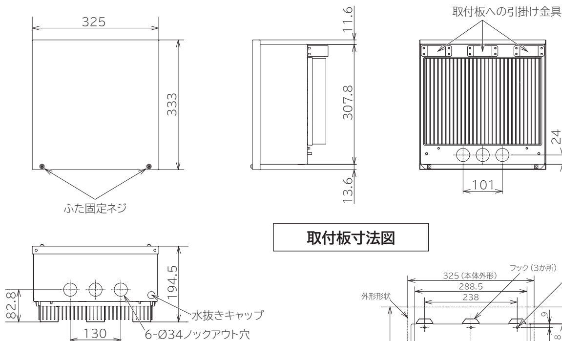
外形寸法図
