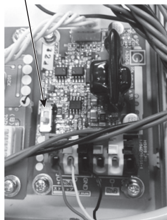
終端抵抗スイッチ
