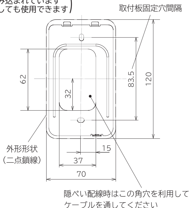
リモコン取付板寸法図
