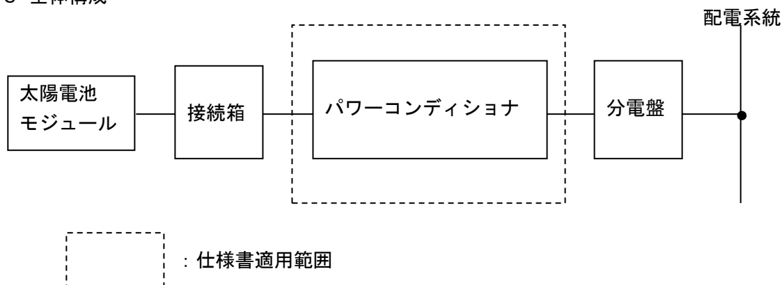
図2-1 全体構成図
