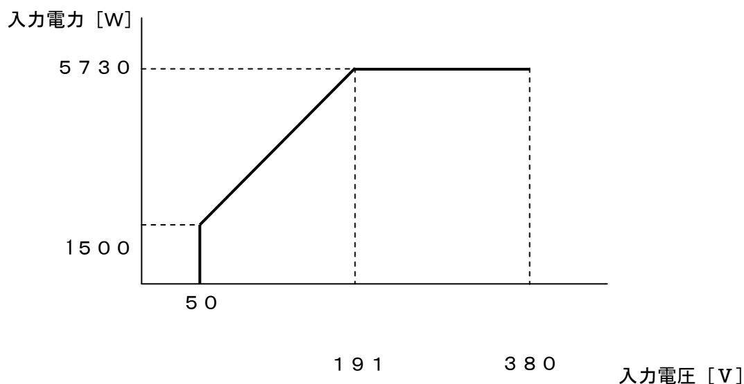
図 3－1 直流入力電圧と入力電力との関係
