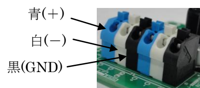
[端子部]
