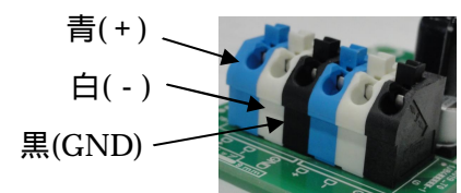
[端子部]
