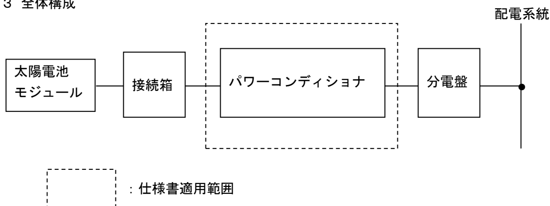
図2-1 全体構成図
