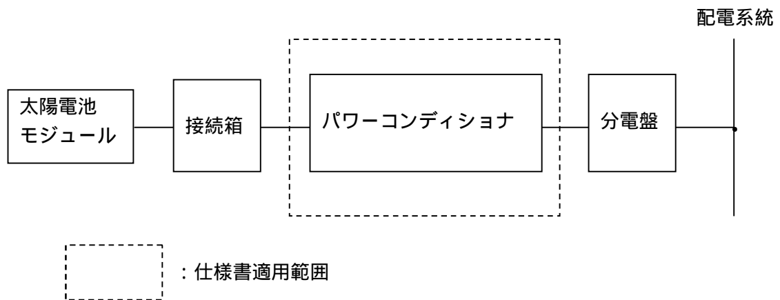
図 2 - 1 全体構成図
