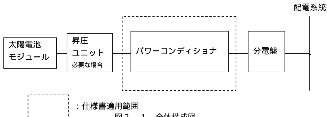
図 2 - 1 全体構成図
