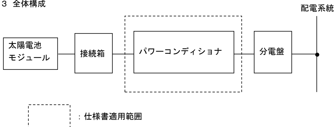
図2-1 全体構成図
