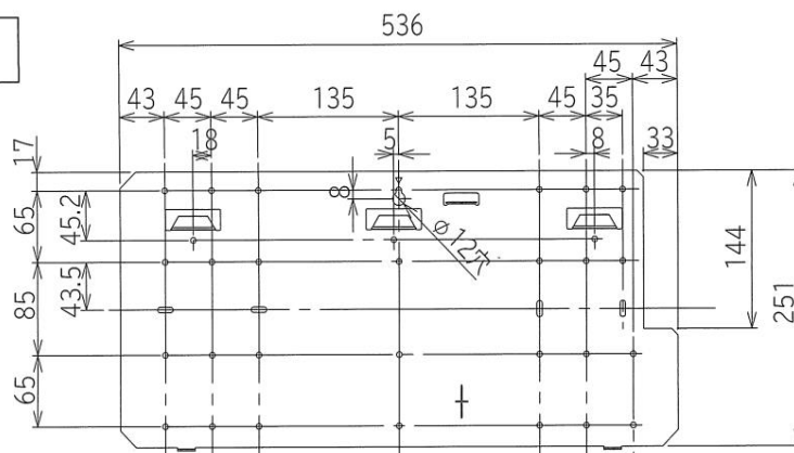
取付板取付穴位置
