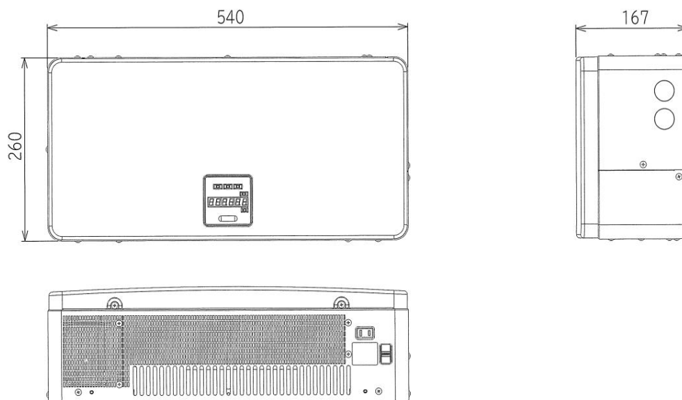
パワーコンディショナ 外形寸法図
