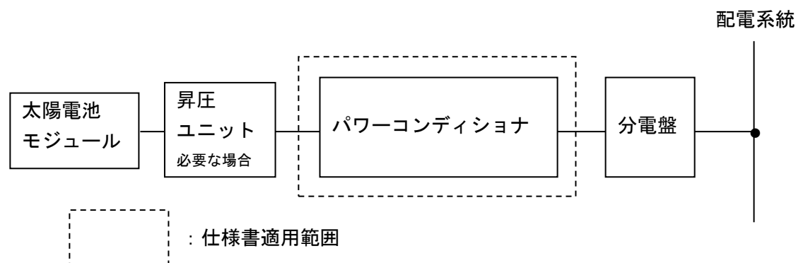
図 2 - 1 全体構成図
