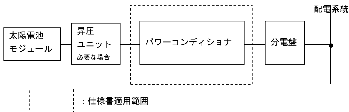
図 2 - 1 全体構成図
