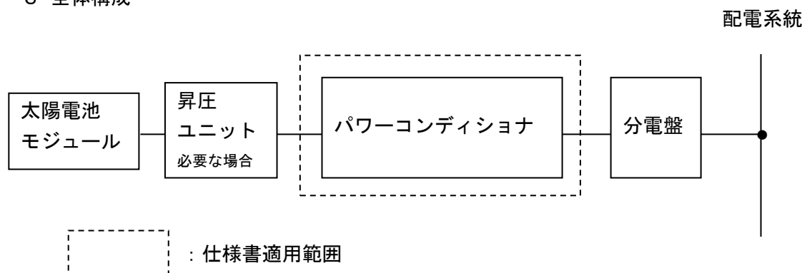
図2-1 全体構成図
