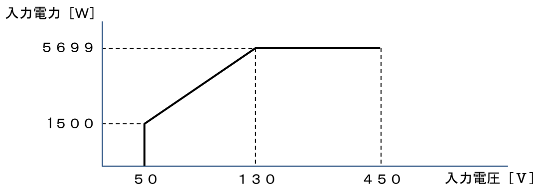
図3-1 直流入力電圧と入力電力との関係
