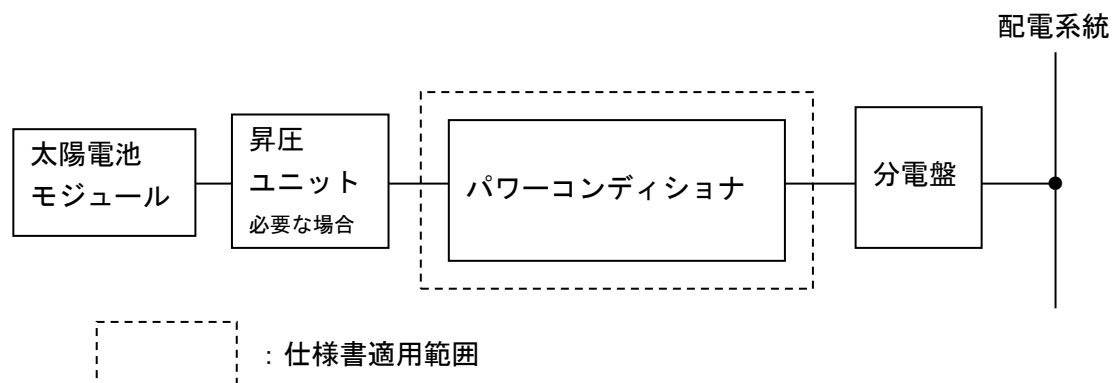
図2-1 全体構成図
