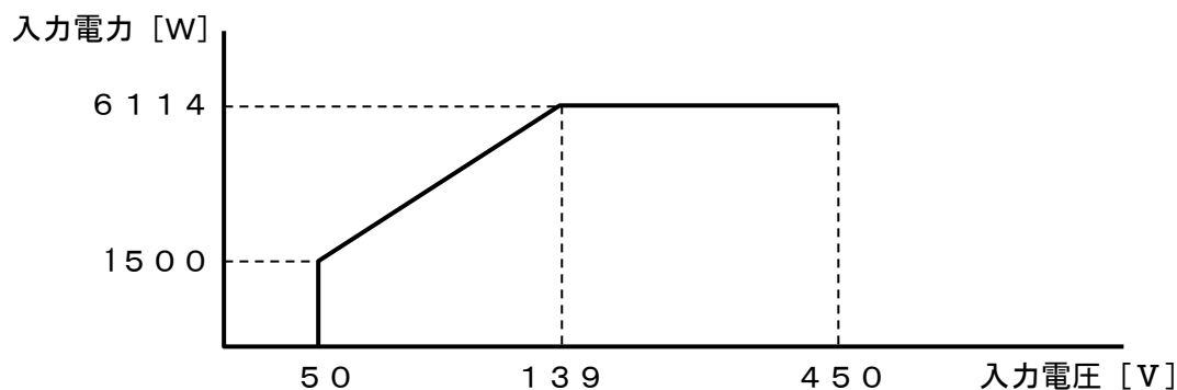
図3-1 直流入力電圧と入力電力との関係
