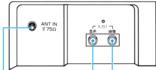
アンテナ端子 (F型コネクター) 音声入力端子 映像入力端子
