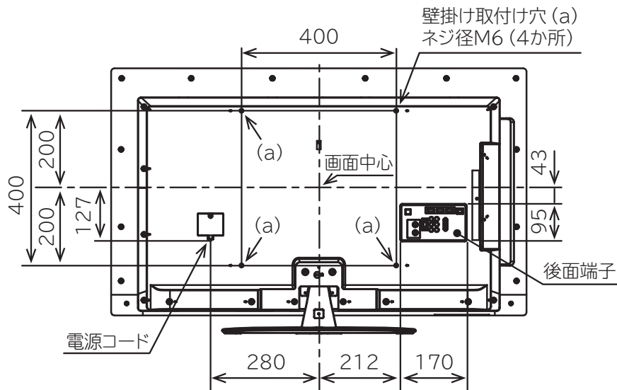
壁掛けユニット(別売)取り付け時の寸法
