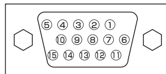
ミニ D-Sub15 ピンコネクタ
