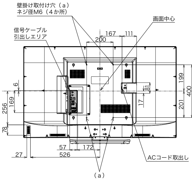
後面図
