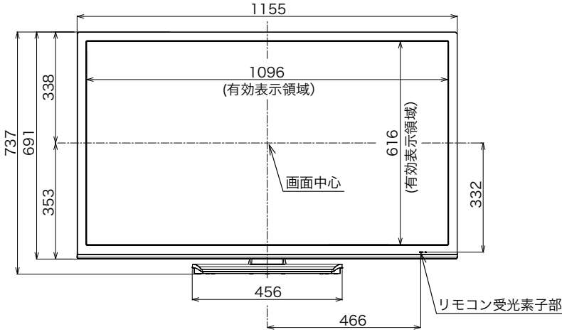
前面図
