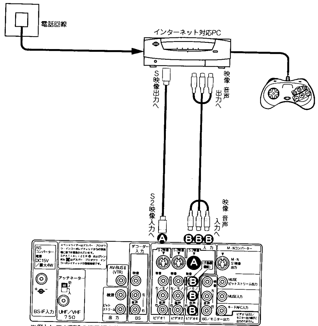
※例として HE72の端子板を使用しています。HE70ご使用の場合、端子の位置が多少異なります。
