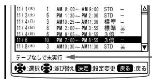
実行結果
