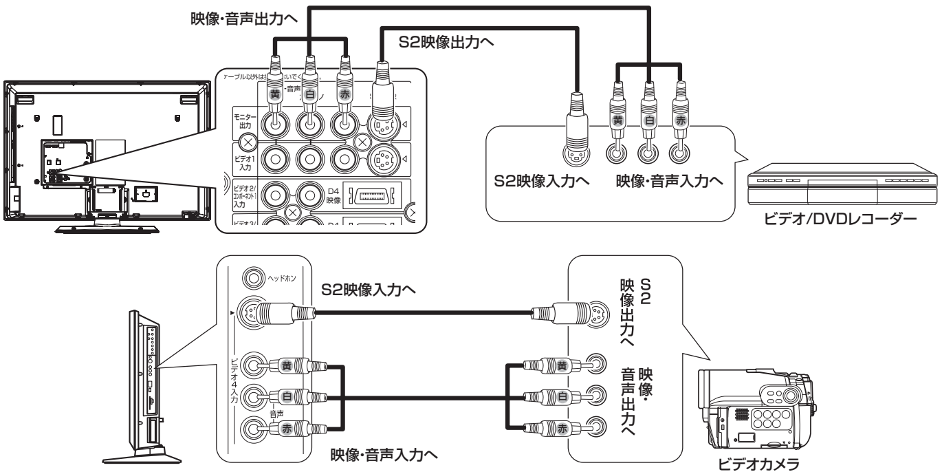
P42-HV01は本体前面に端子があります。
