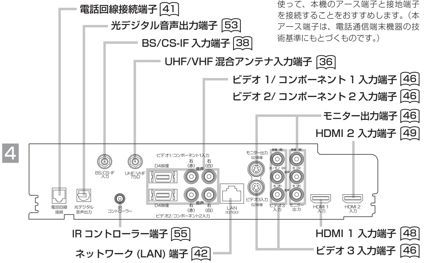
後面端子 端子の捺印は、端子の下にあります。
