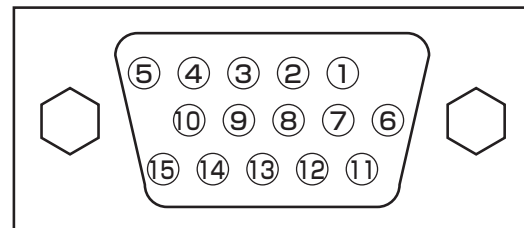
ミニ D-Sub15 ピンコネクター
