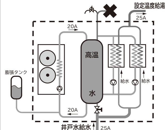
井戸水使用の給湯サイクル図（イメージ図）
