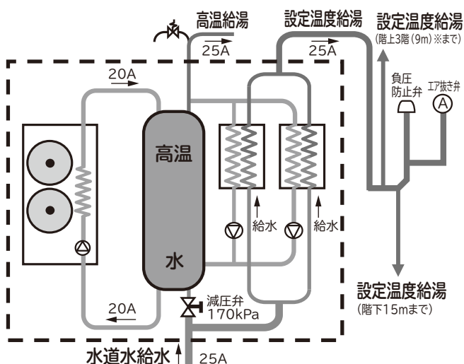
階下・階上給湯サイクル図（イメージ図）
