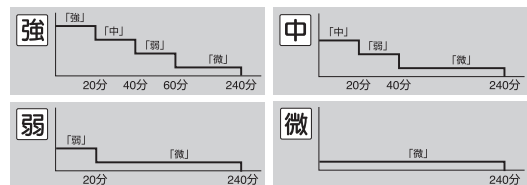
風量設定ごとの風量の下がり方(切タイマー4時間設定の場合)
