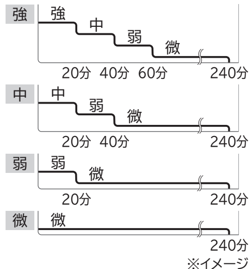
風量設定ごとの風量の下がり方 (設定例: 切タイマー4時間設定の場合)
