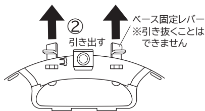
ベース裏面
