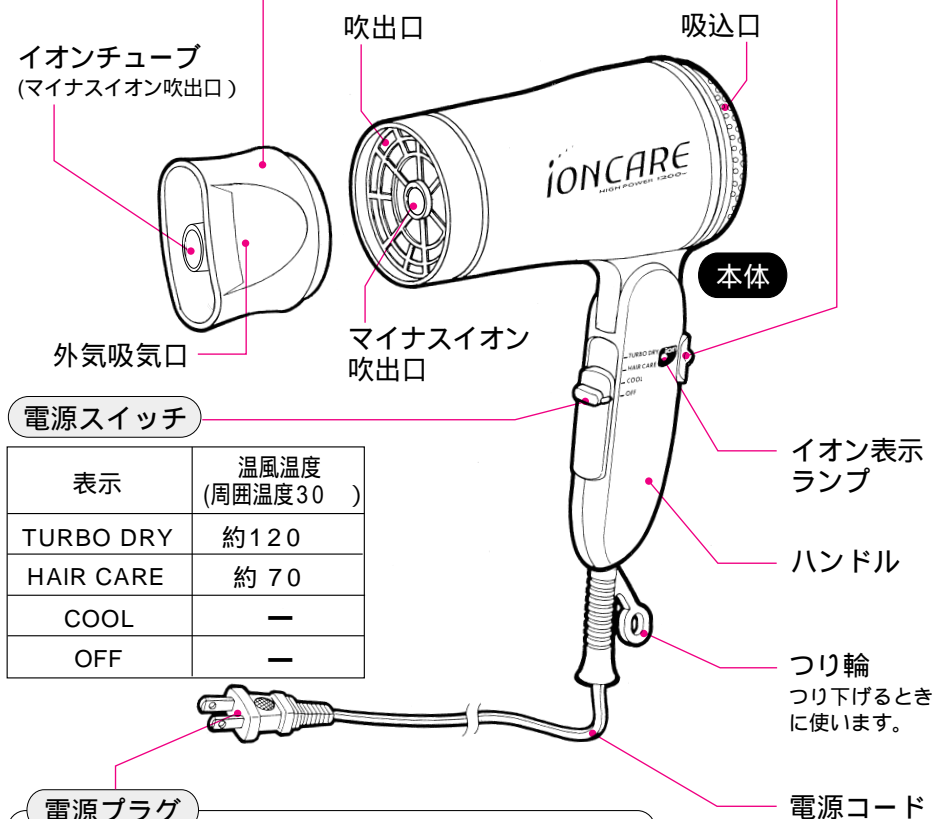
電源プラグ
