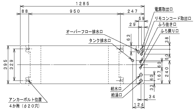
配管取出し位置図
