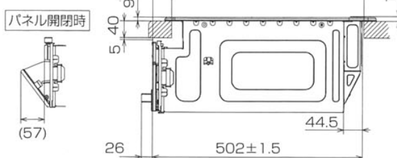
側面図
