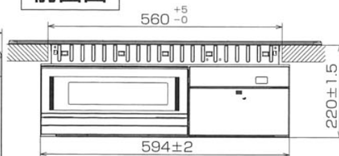
前面図
