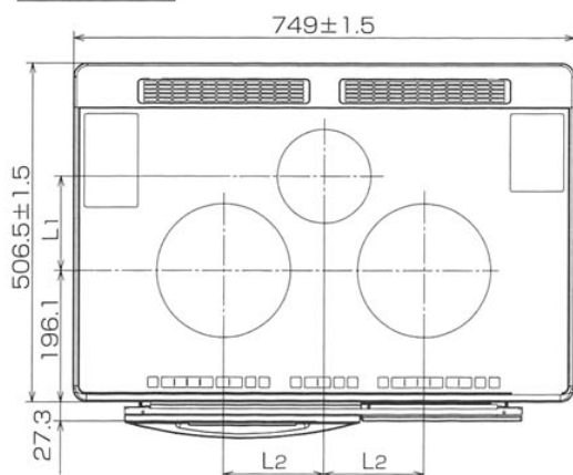
上面図
