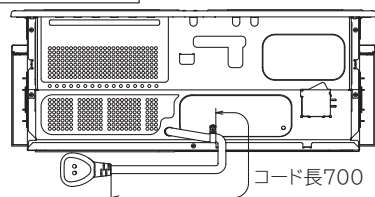
後面図
