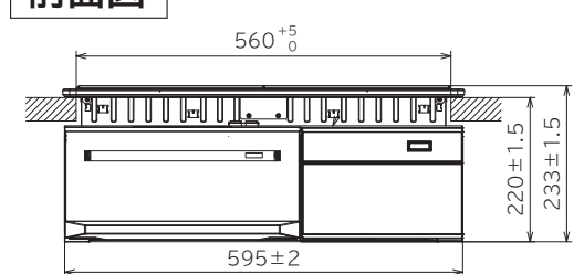
前面図
