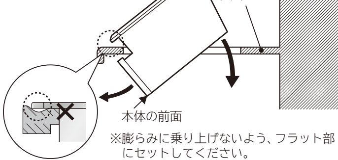
断面図
