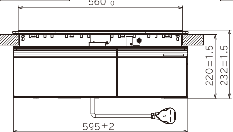
前面図
