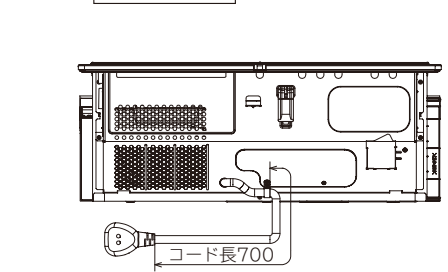
後面図
