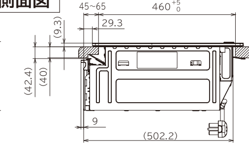
側面図
