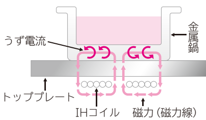
IH加熱の原理(イメージ図)
