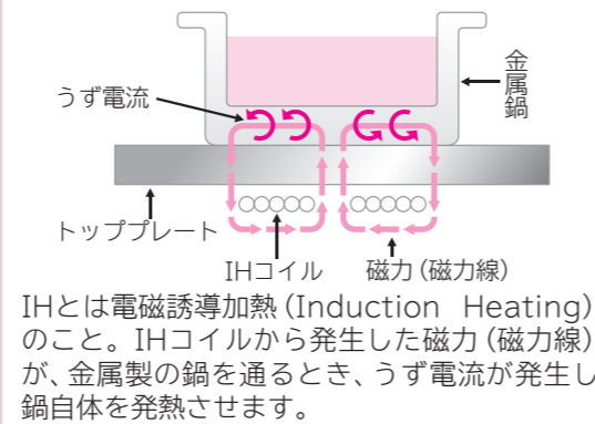
IH加熱の原理(イメージ図)
