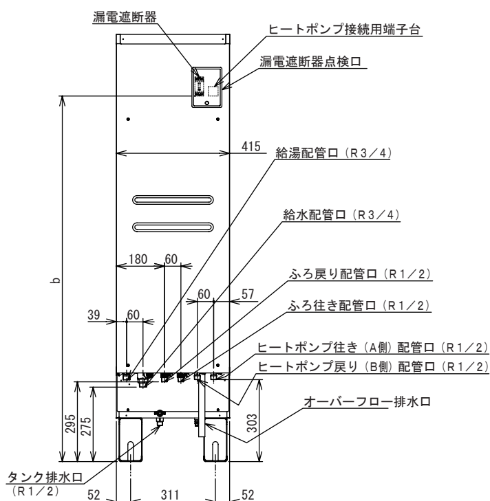
貯湯ユニット脚部寸法
