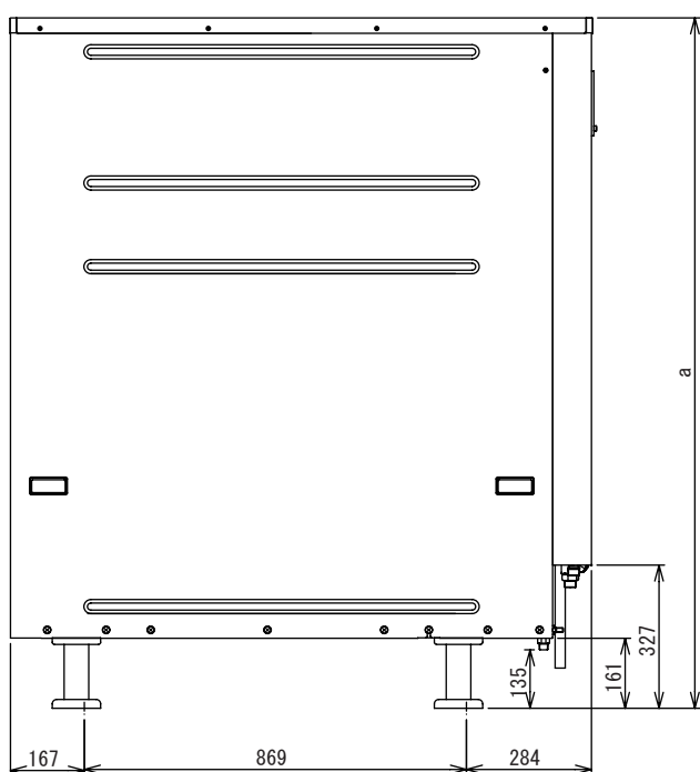
配管取り出し位置図
