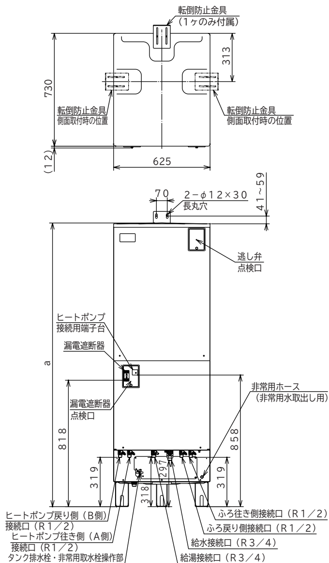
配管取り出し位置図
