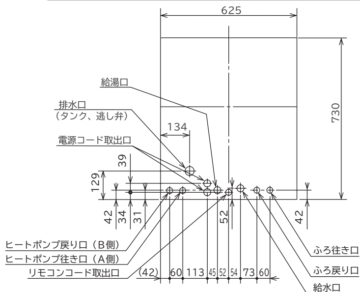
配管取り出し位置図
