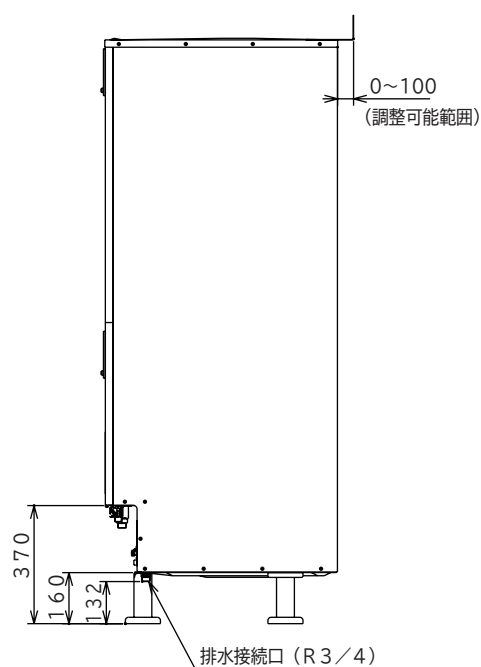
貯湯ユニット脚部寸法
