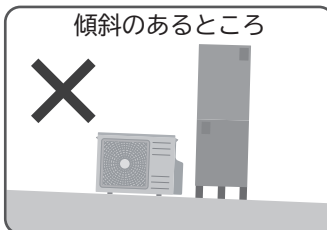
水平な設置面に垂直に立てて据え付けてください。 (傾斜許容限界2/100)
