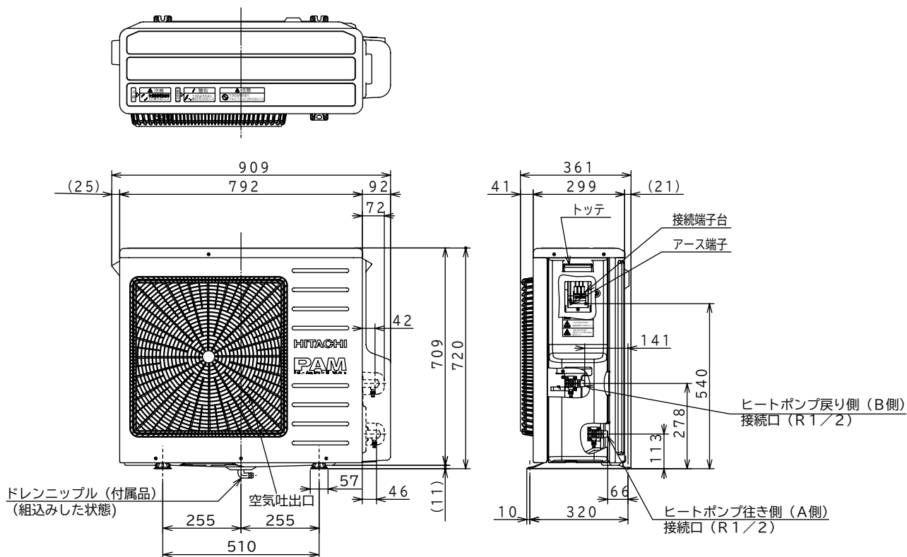
ヒートポンプユニット (BHP-HAV60L、BHP-HAV45L、BHP-HA60L、BHP-HA45L)
