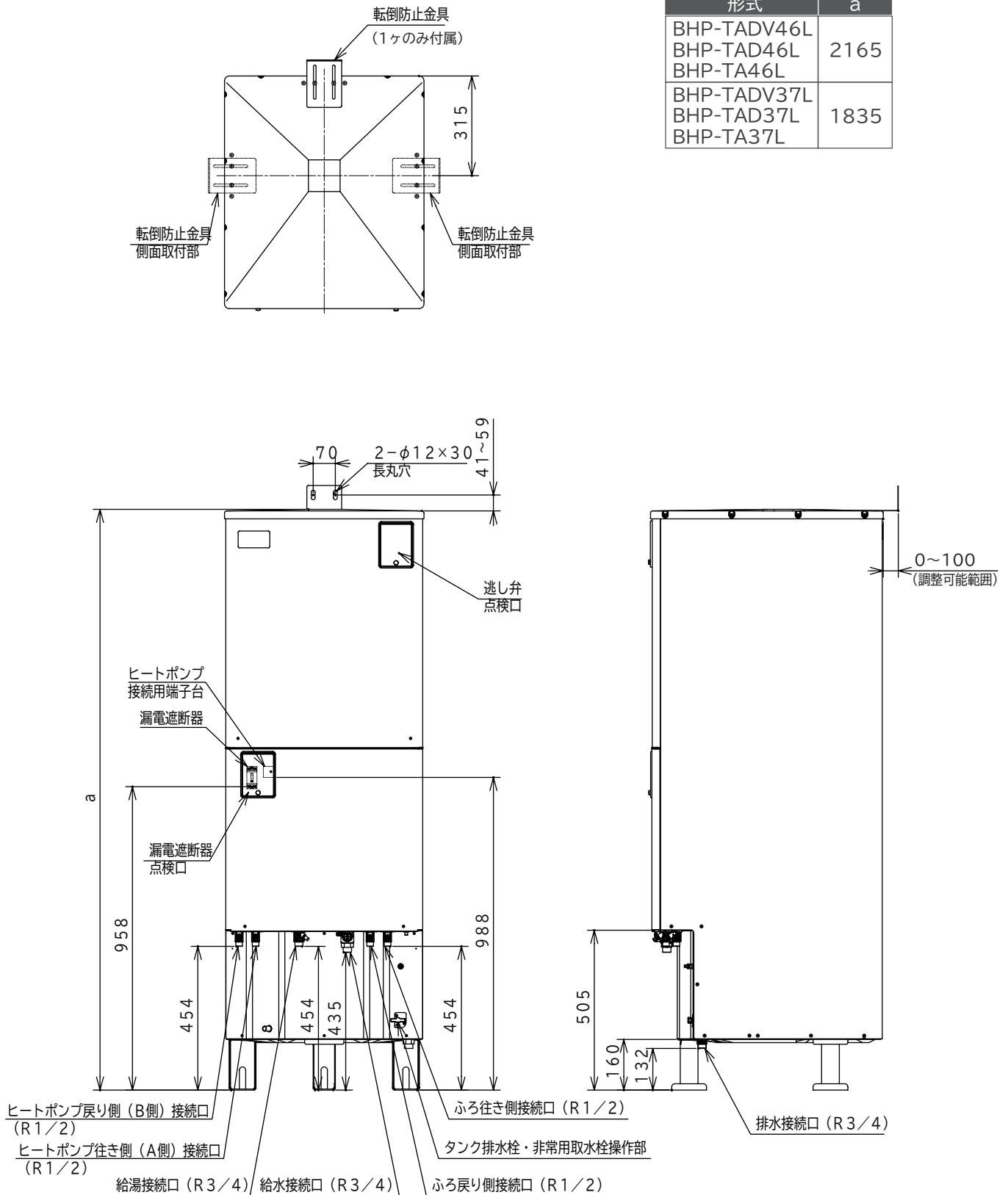
貯湯ユニット
