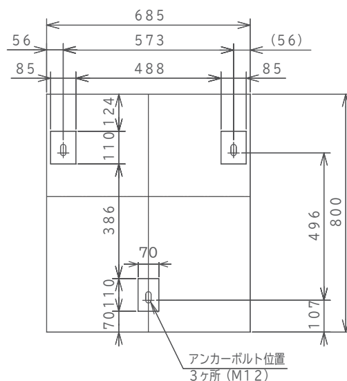
貯湯ユニット脚部寸法
