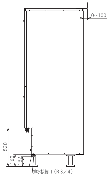
貯湯ユニット脚部寸法
