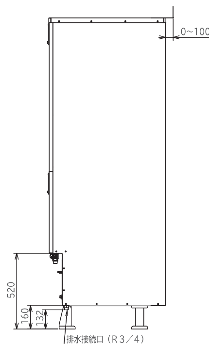
貯湯ユニット脚部寸法
