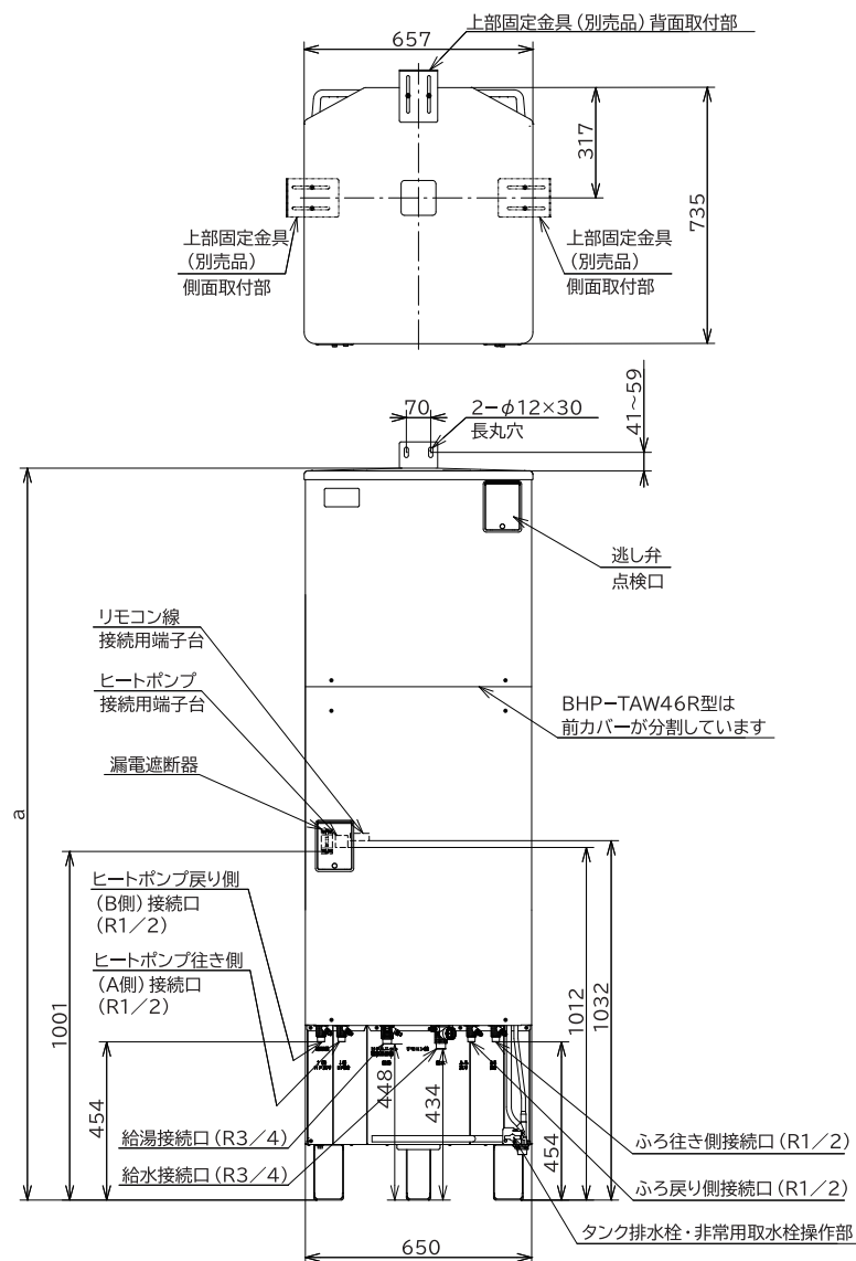
配管取り出し位置図
