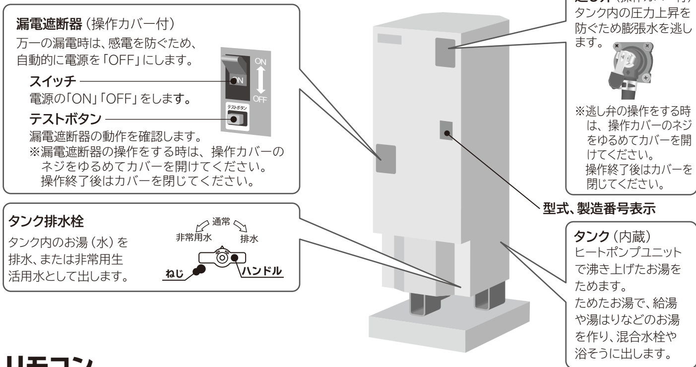
貯湯ユニット(タンク)
