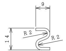
A - A 断面図
