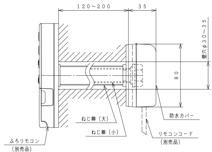
防水カバー、ねじ棒 (大) (小) 取付図
