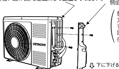
RAC-AJS25Z・AJS28Z・AJS36Z
