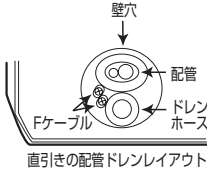
直引きの配管ドレンレイアウト
