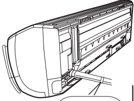
Fケーブル、配管、ドレンホースをテープ止めます。
