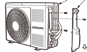
RAC-AN28C
